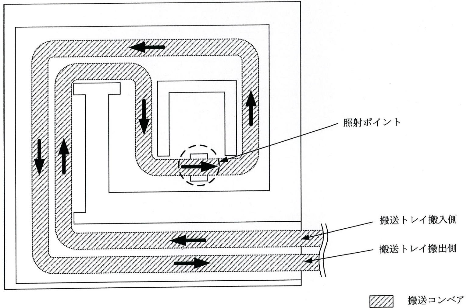
照射室内図（電子線照射施設1F）
